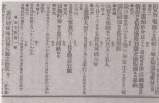
图13 1910年(清宣统二年)10月19日《申报》对运动会的报道
