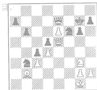
30. ♕a3!!
