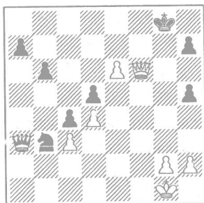
34. e7
