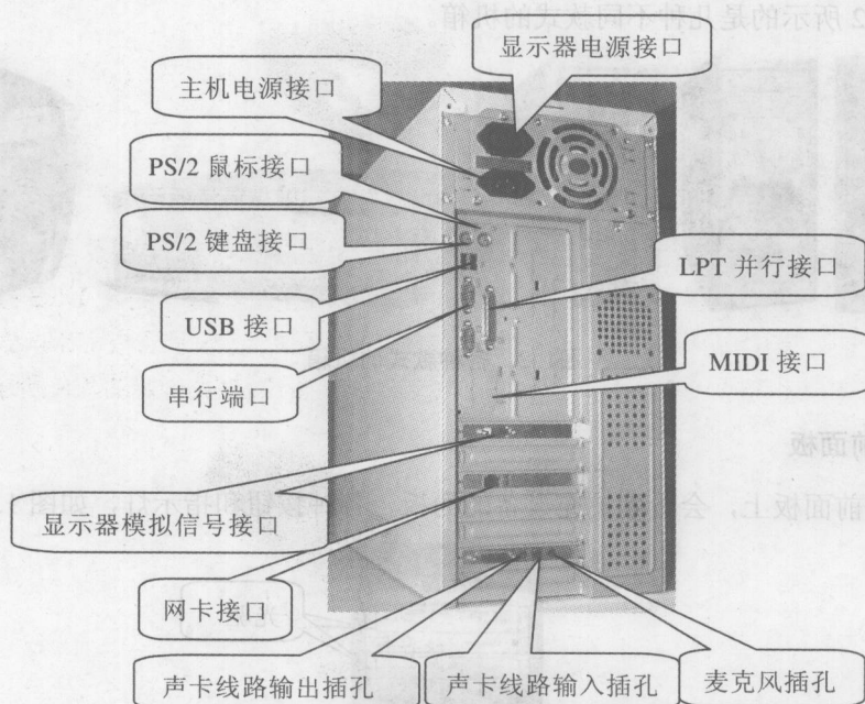
图1.4 主机背面板
