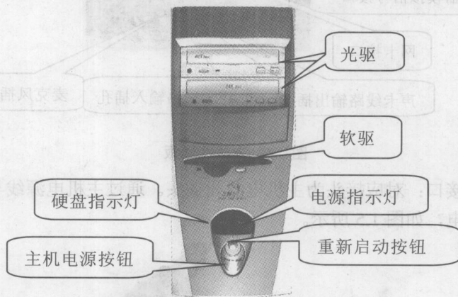
图1.3 典型的主机前面板
