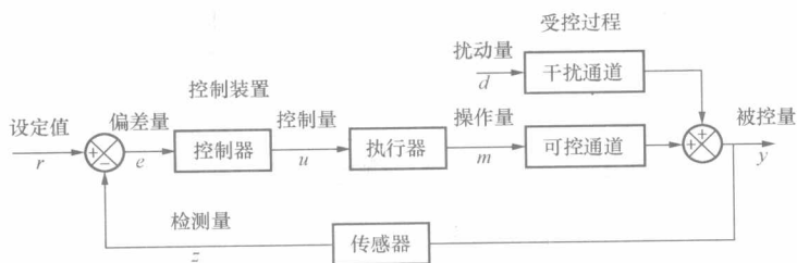
图 1-3 反馈控制系统方框图
