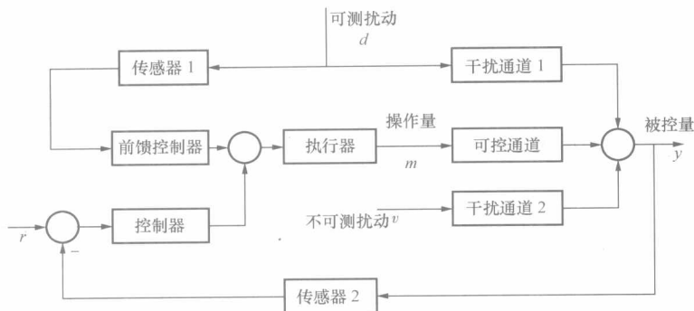
图 1-9 前馈—反馈复合控制系统方框图
