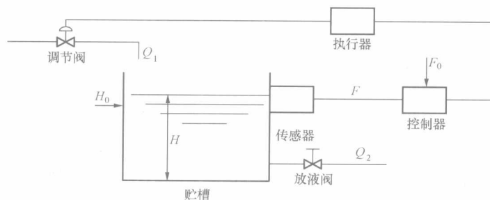
图 1-2 贮槽液位控制系统的原理结构图
