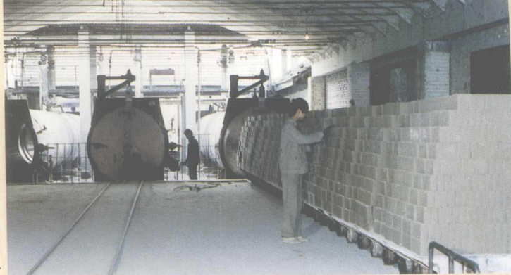
内江市建材化工厂灰砂砖生产车间
