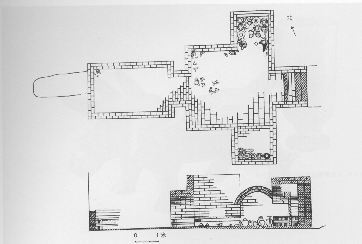
● 5.10 洛阳曹魏正始八年墓平、剖面图
