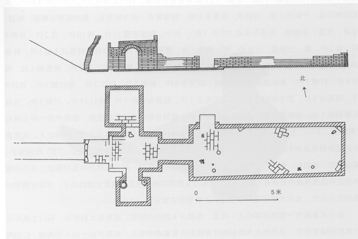
● 5.12 杏园6号墓平、剖面图
