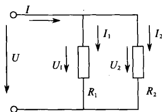
图 1—6 两个电阻并联的电路
