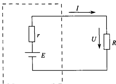
图 1—4 全电路
