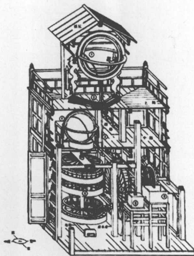
水运仪象台结构图
