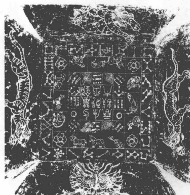
南唐墓盖上的二十八宿。1964年出土于江苏邳江墓中。墓盖刻于南唐大保四年(946)。墓盖顶部内刻日、月、华盖(杠)和勾陈星宿、八卦,中部刻十二生肖,外刻二十八宿,墓盖四面刻有四像之神,即苍龙、白虎、朱雀、玄武。
