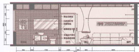
C立面图
