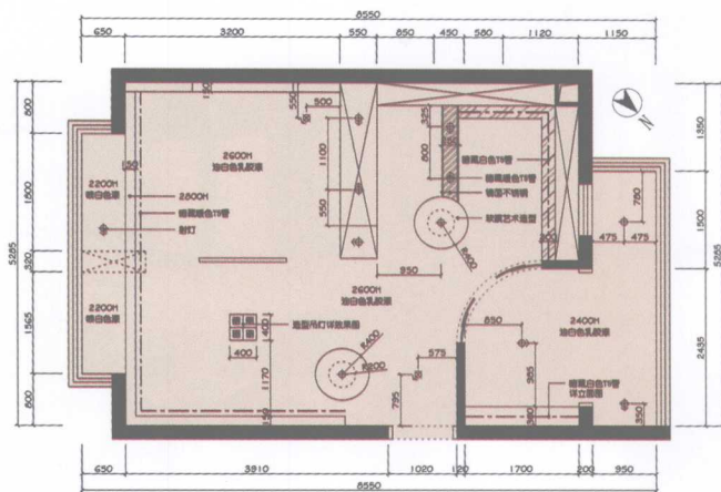
⊙ 天花灯位图
