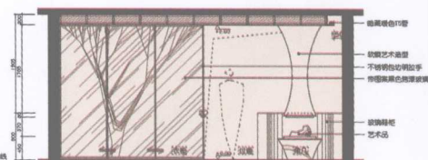
B立面图
