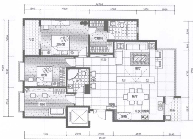
◎ 平面布置图
