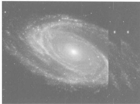
星系
