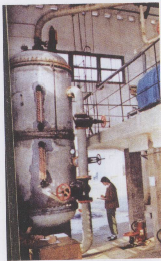
丰顺县邓屋地区建成我国第一座地热试验电站。图为电站一角。
