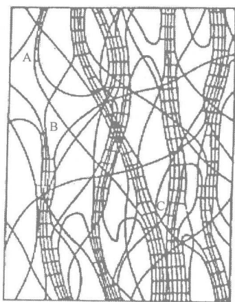
图 1-7 Hearle 的缨状原纤结构
