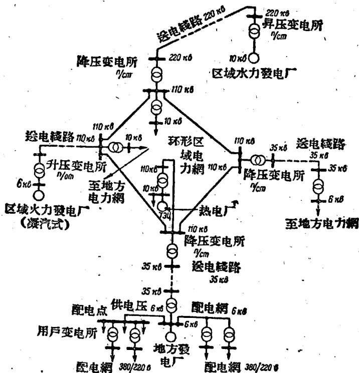
圖 1-1 电力系统圖
