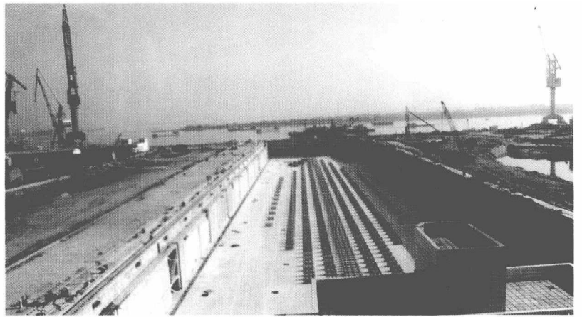
► 文冲船厂1995年3月建成的15万吨级干船坞
