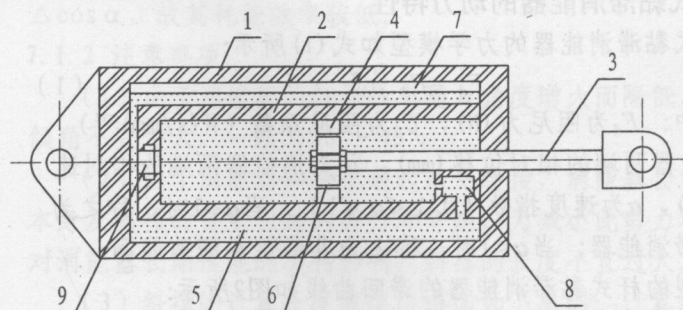
1-外缸 2-内缸 3-导杆 4-活塞 5-阻尼材料 6-阻尼孔 7-储油箱 8-拉伸压缩调压阀 9-底部检验孔
