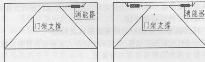
(b) 正门架双侧型
