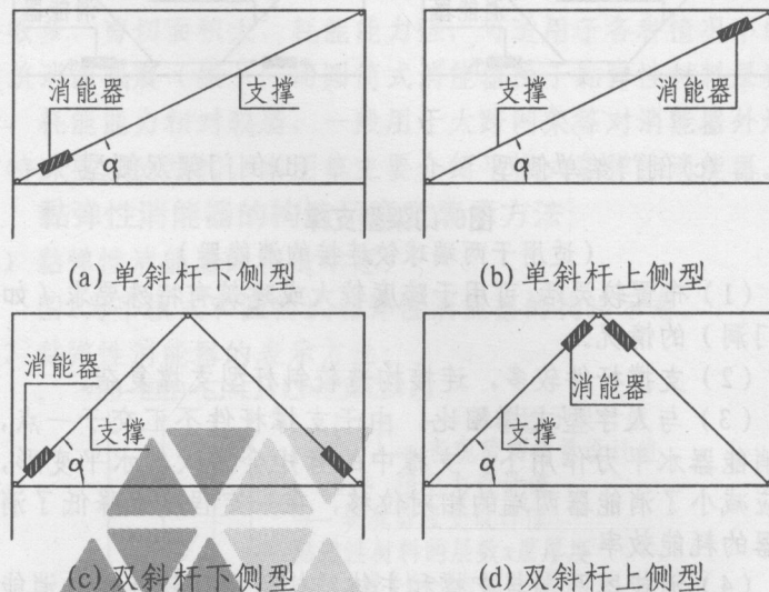
图4 斜杆型支撑
