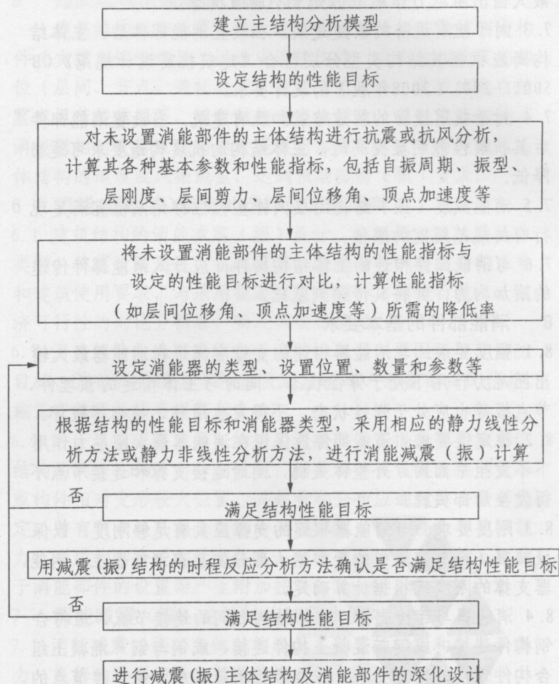
图10 消能减震(振)结构的计算流程
