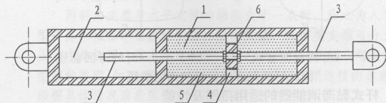
1-主缸 2-副缸 3-导杆 4-活塞 5-阻尼材料 6-阻尼孔
