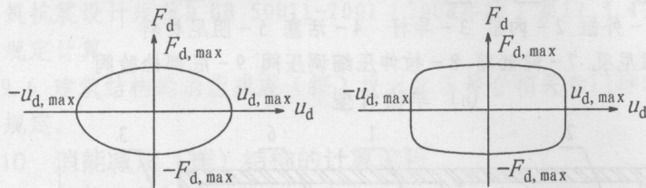
(a) \alpha=1.0 时的滞回曲线 (b) \alpha=0.4 时的滞回曲线
