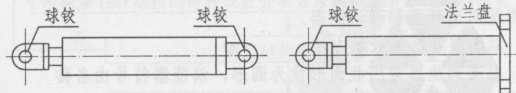
(a) 两端球铰连接 (b) 一端球铰连接一端法兰连接
