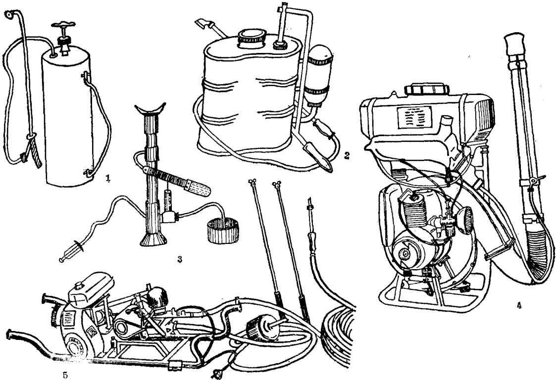
图1 各种喷雾器
