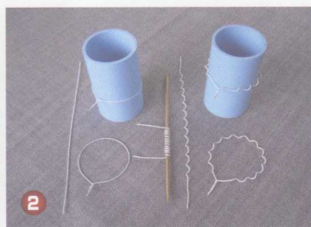
2. 曲线线圈是在套筒绕制前用竹针绕曲后加工而成的。
