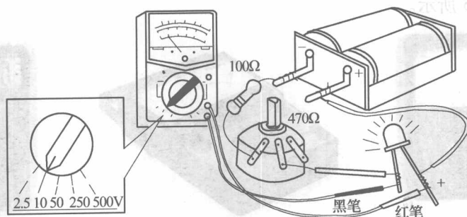
图 1-2-6 用万用表测电压接线图
