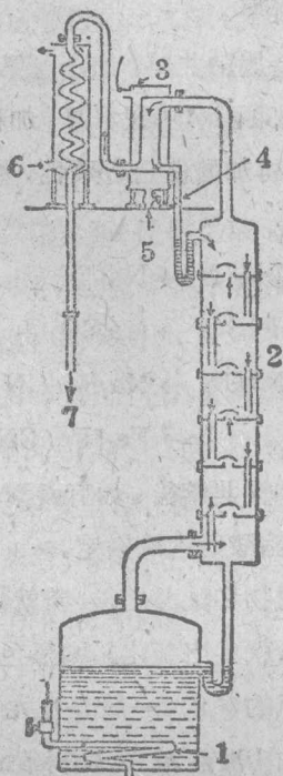
圖2 工業上用的蒸餾鍋和分餾塔
