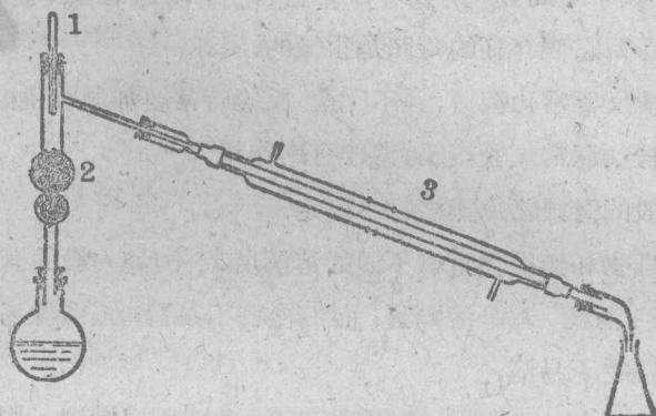
圖1 實驗室分餾裝置
