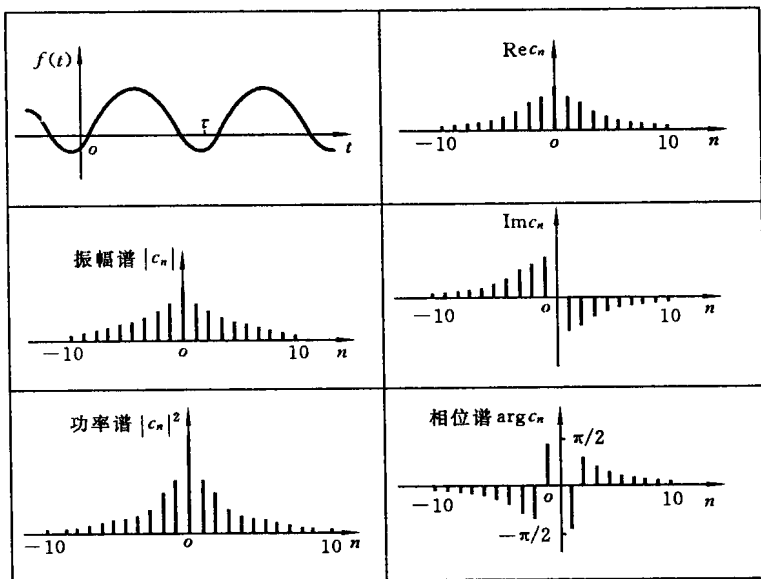
图 1.1 Fourier 级数频谱示意图
