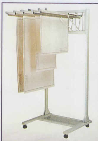
转拉式图纸架 铝合金 A0 图纸夹 6 小支架 6 储物网 1 W: 680 D: 960 H: 1490
