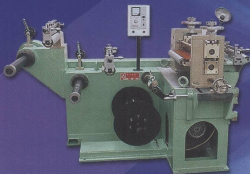
钢带分切设备(系列产品)
