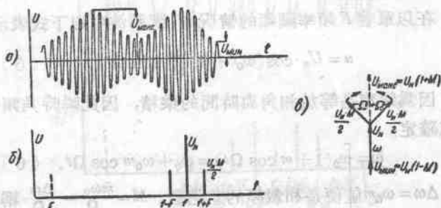
圖2. 調幅振盪
