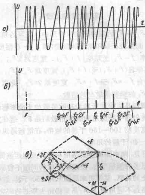
圖3. 調頻振盪
