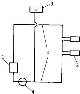
图 0-1 集中式热水供暖系统示意图
