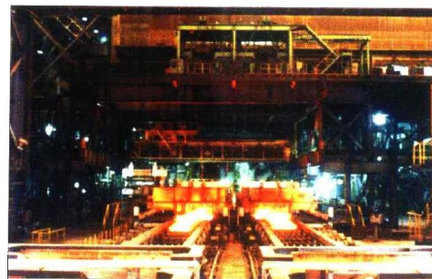
1450mm板坯连铸机
