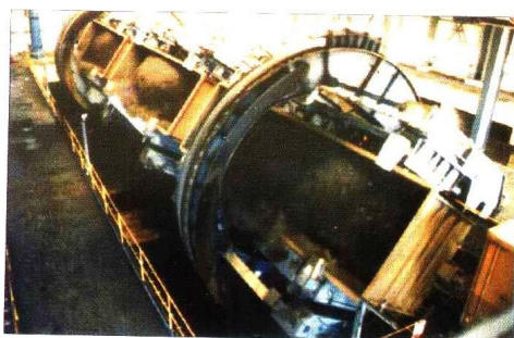
三车翻车机
