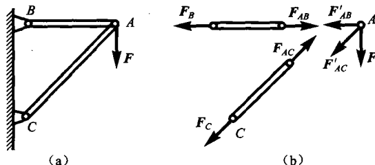
图 1-5 作用力与反作用力 (a) 杆件受力 F ; (b) 受力图
