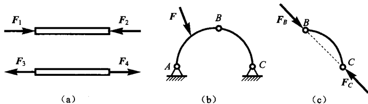
图 1-1 二力构件
