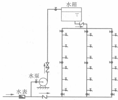
图 1-12 环状网给水方式
