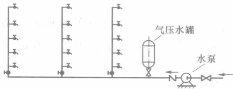
图 1-11 设气压供水装置的给水方式
