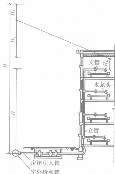
图 1-2 建筑内给水系统所需压力示意图
