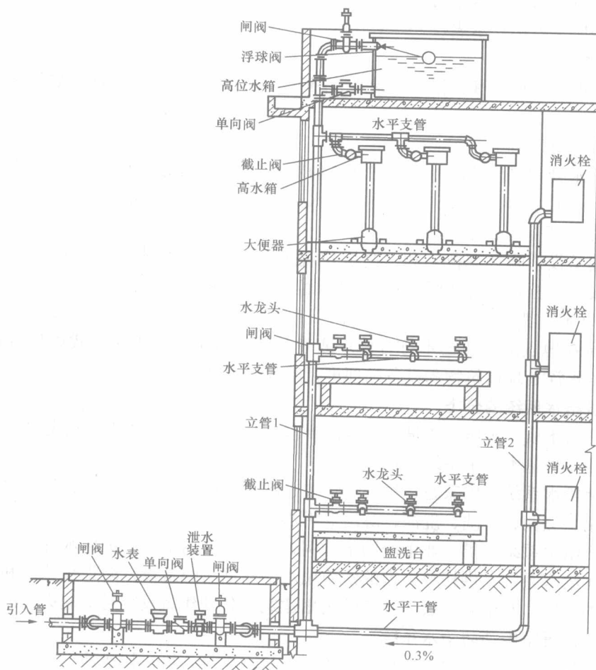
图 1-1 建筑给水系统的组成
