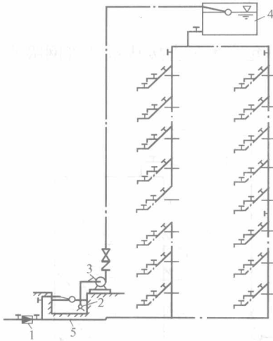
图 1-10 分区、分压的给水方式
