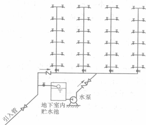
图 1-7 水泵从断流水池吸水示意图
