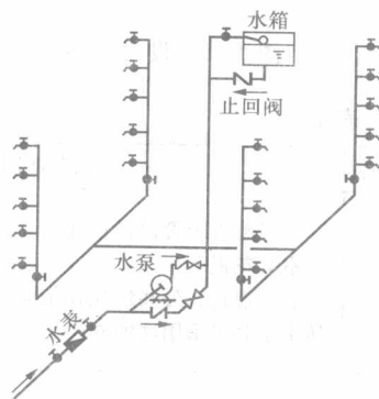
图 1-9 设水泵和水箱联合工作的给水方式
