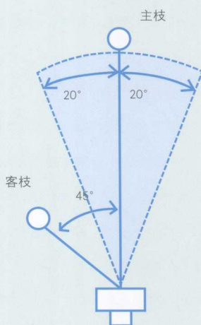
侧面图
