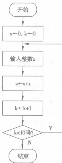
图 1-2 输入 10 个整数求和计算的算法
