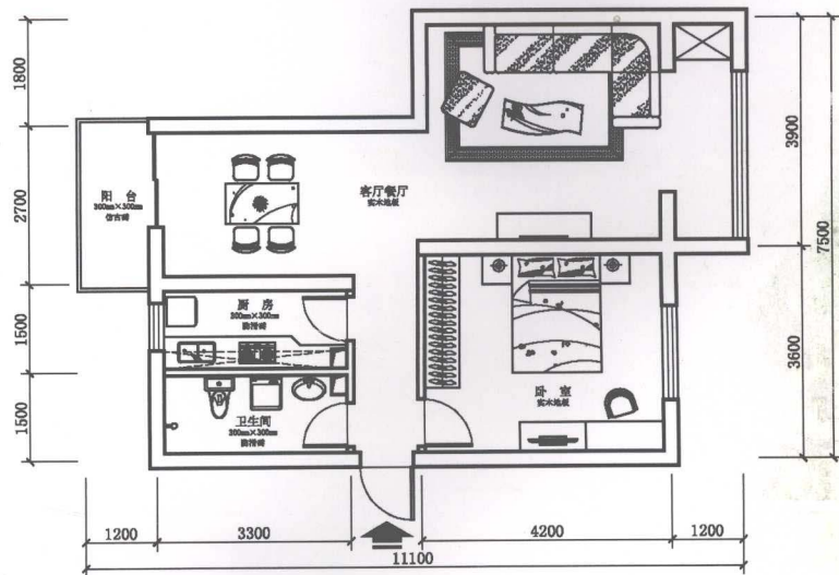
▲ 平面布置图
