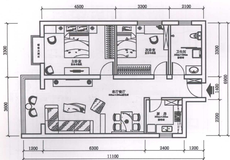
▲ 平面布置图
