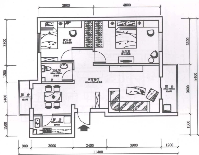
▲ 平面布置图
