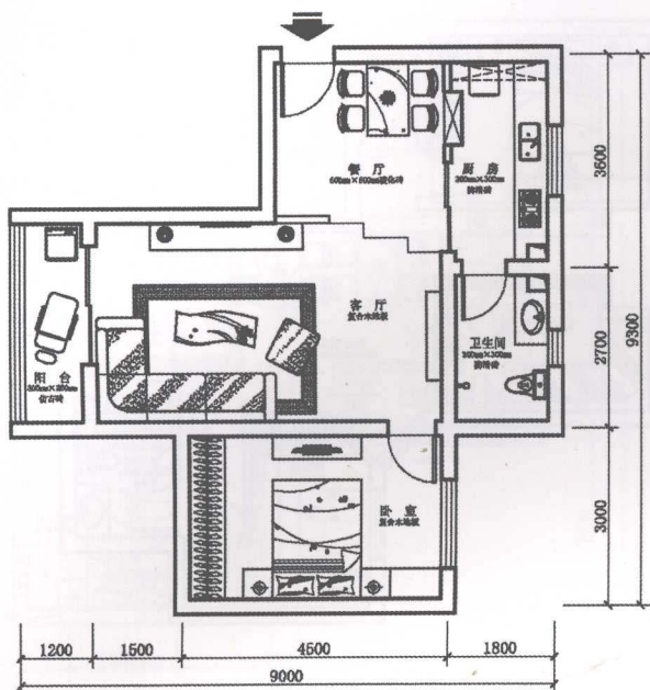
▲ 平面布置图
