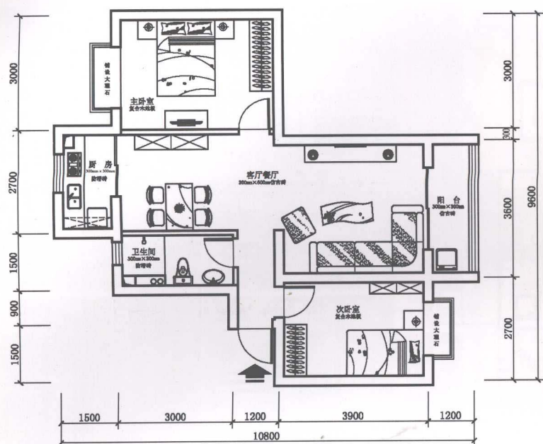
▲ 平面布置图
