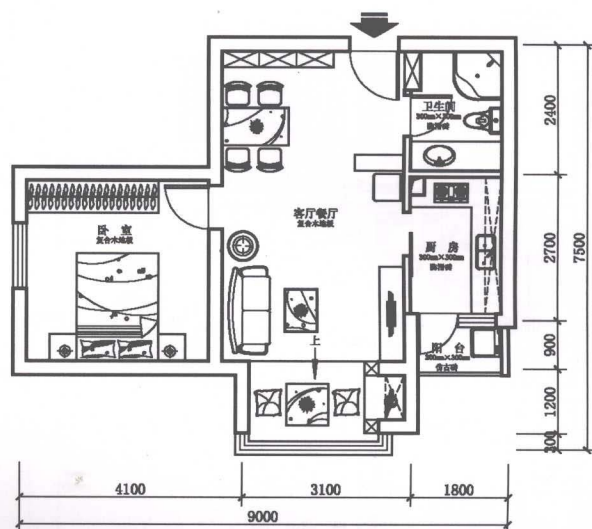
▲ 平面布置图
