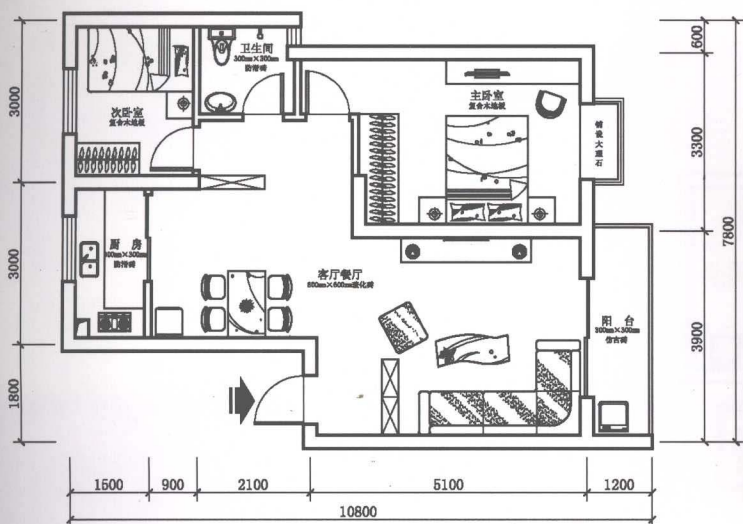
▲ 平面布置图
