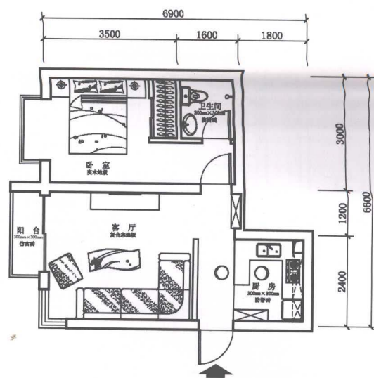
▲ 平面布置图
