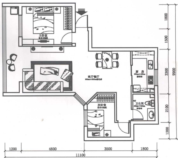
▲ 平面布置图
