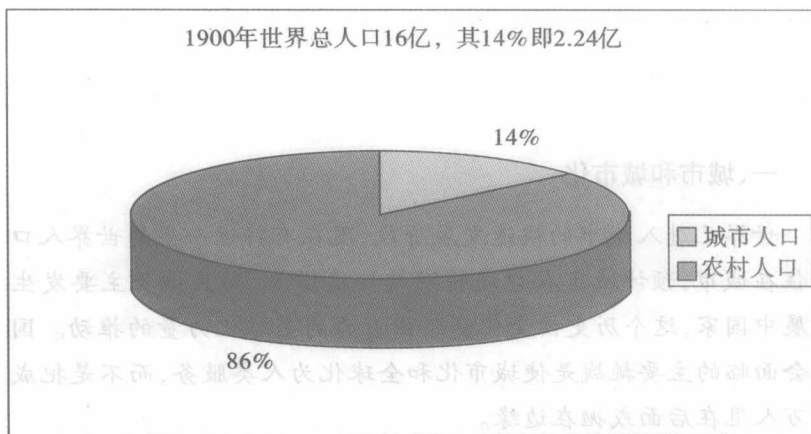
城市人口占全球总人口的比例(1900 年)
