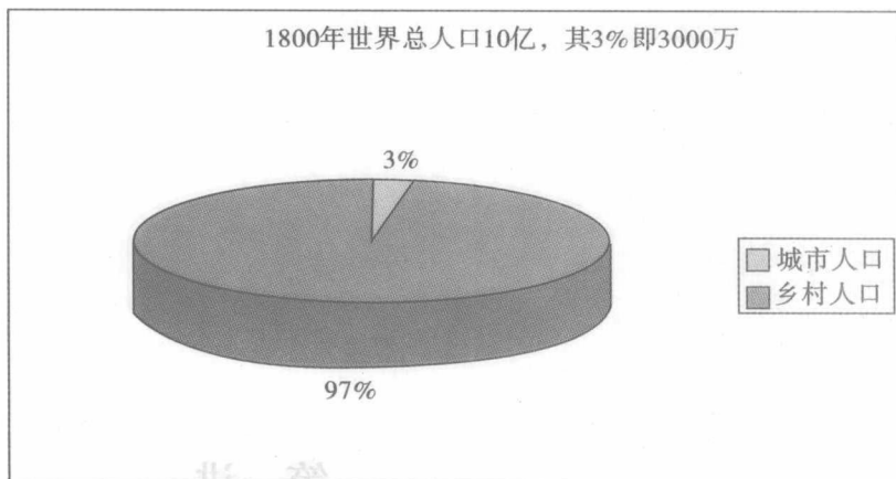
城市人口占全球总人口的比例(1800 年)
