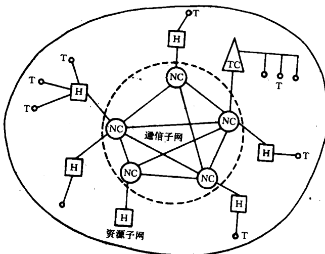
图 1-3 计算机网络的构成
