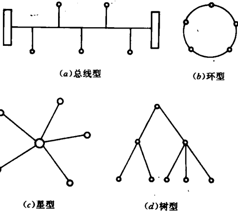
图 1-8 局部网网络拓扑结构
