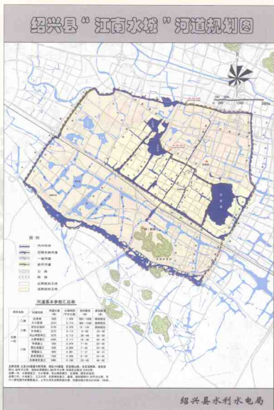
绍兴县“江南水城”河道规划图。
