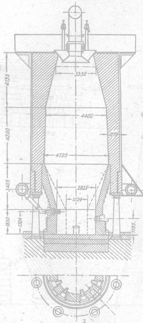
圖例 2. 爐身放置在支柱上的輕裝煉鐵爐。 ■ 1——英國克拉朗斯廠 ■ 2——唐柏斯地方的蘇令斯基廠 ■ 3——賓夕爾凡尼亞地方用無烟煤的煉鐵爐
