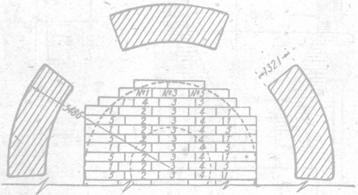
窩底平面圖
