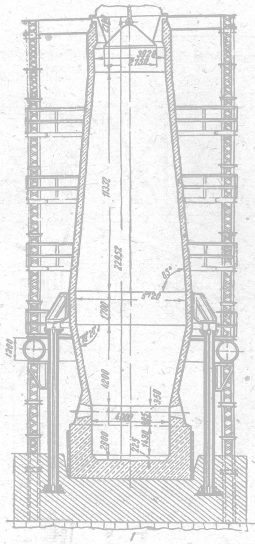
圖例 12. 薄壁爐身的煉鐵爐。 ■ 1—依里諾斯公司的煉鐵爐 ■ 2—哥索高爾斯基廠的煉鐵爐 ■ 3—捷克斯拉夫的克拉達諾廠煉鐵爐
