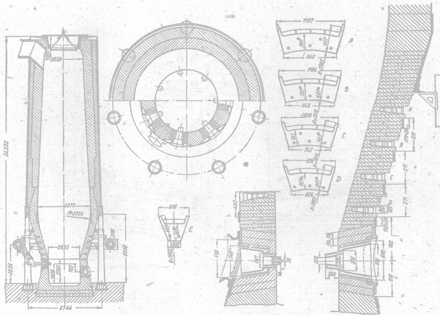
圖例 6. 賓夕爾凡尼亞地方恩杜佛廠的煉鐵爐。
