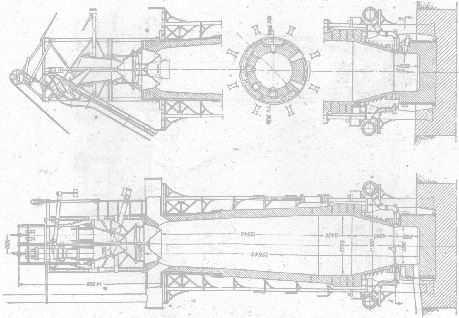
圖例10. 克刺馬安斯基廠的煉鐵爐。
