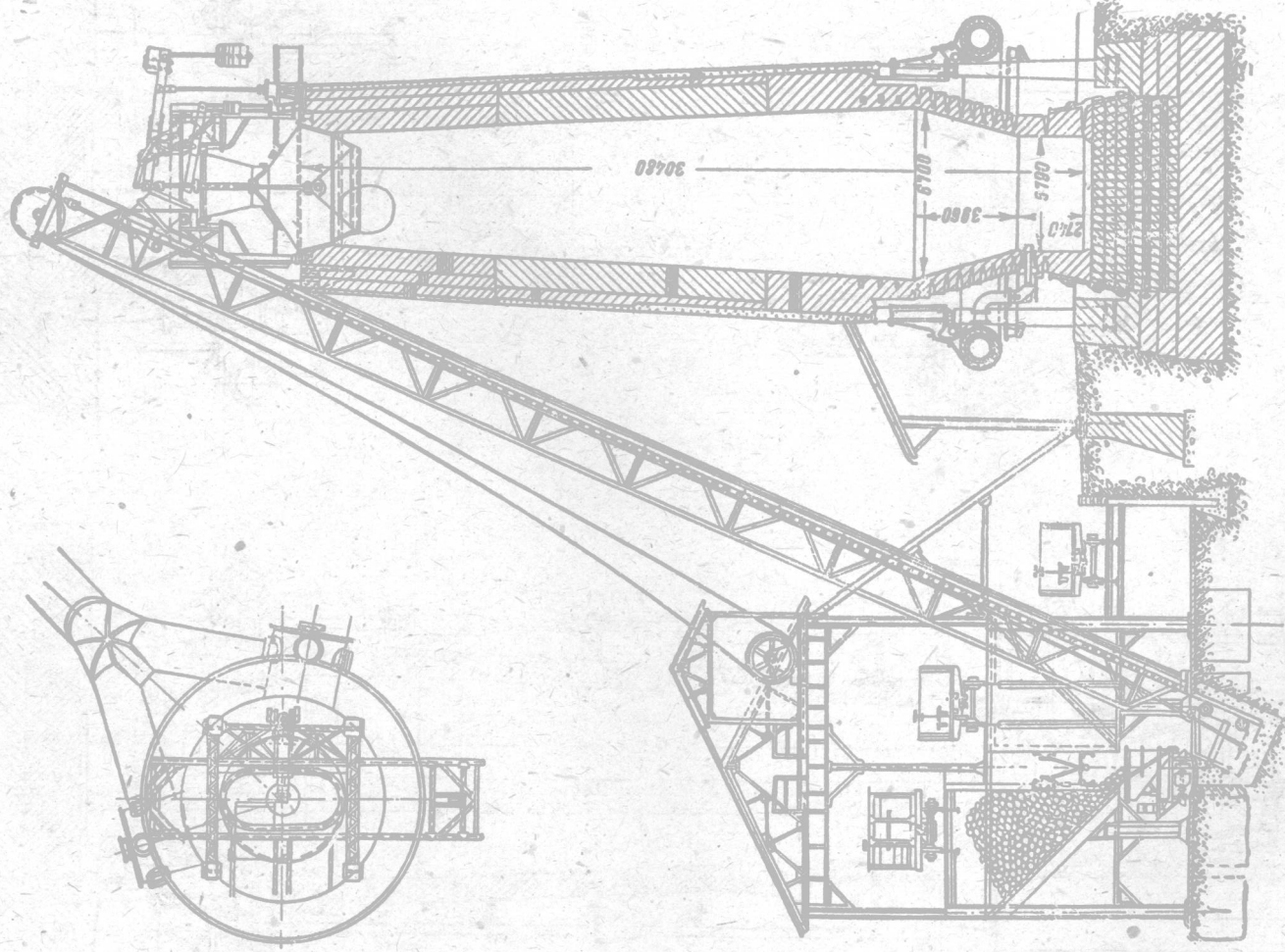
圖例 9. 美國依雷斯的焦炭煉鐵爐
