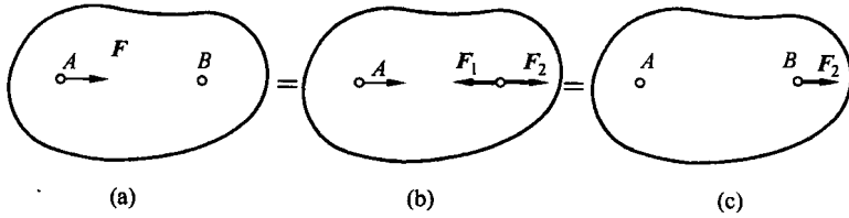
图 1.6 力的可传性
