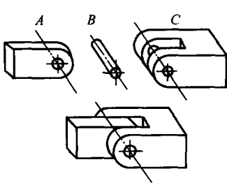
图 1.12 铰链连接
