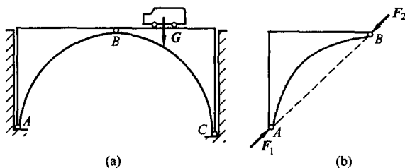
图 1.4 二力构件
