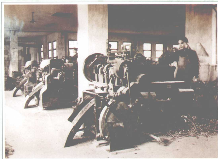
贵阳市卷烟工业使用的 第一代上下式切丝机
