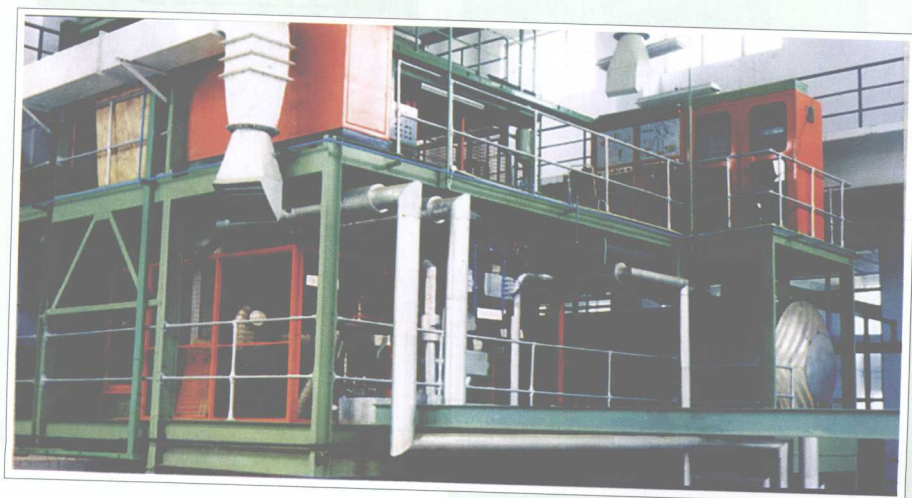
贵阳卷烟厂二氧化碳膨胀烟丝线
