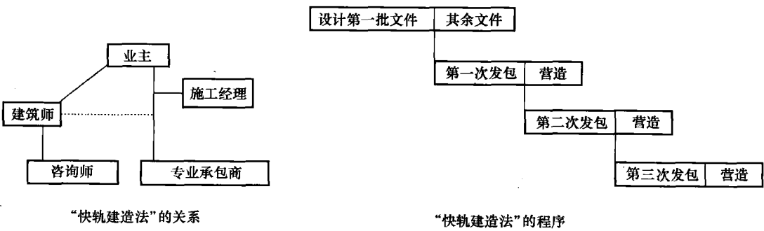
图 1-2 快轨建造法
