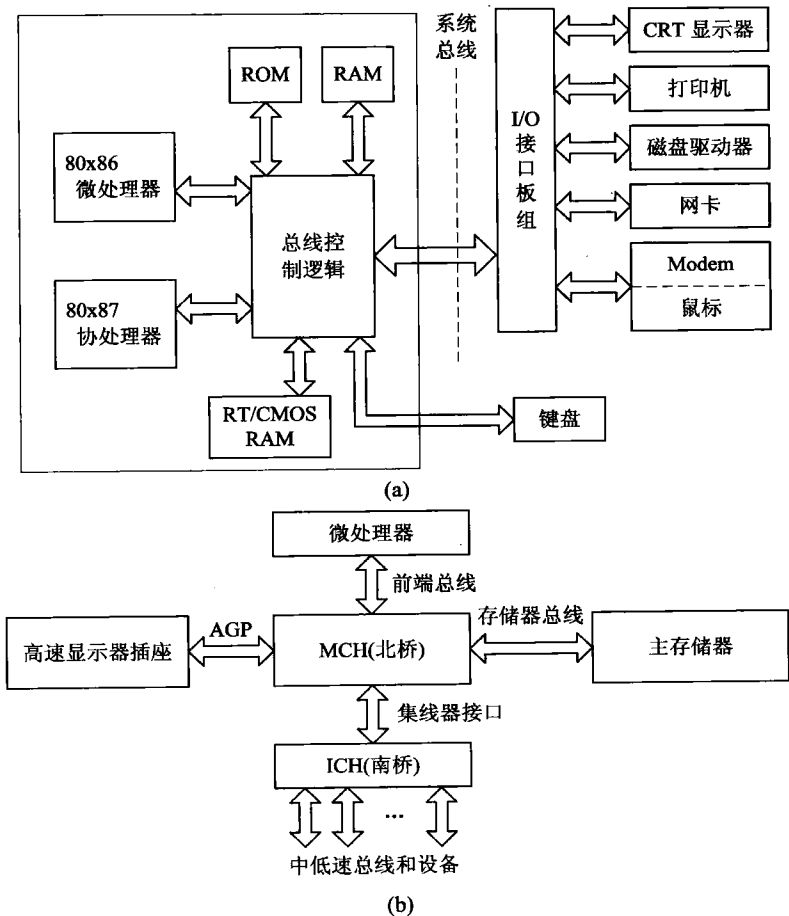
图 1.1 微机系统硬件组成框图
