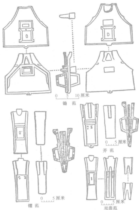
图二 河北兴隆发现的战国生产工具铸范
