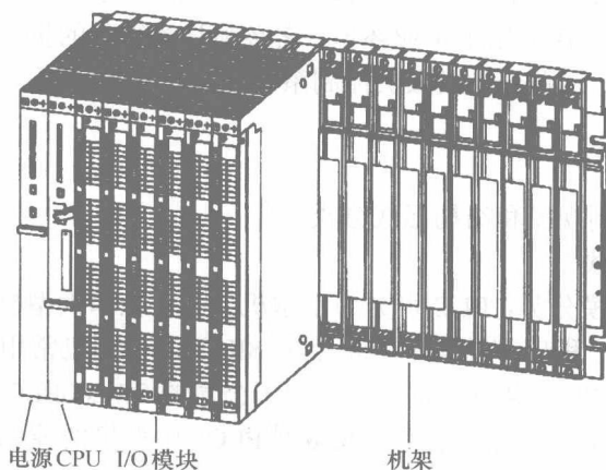
图1-3 模块式S7-400PLC
