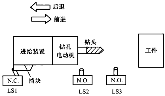
图1-1 进给装置的逻辑控制顺序图
