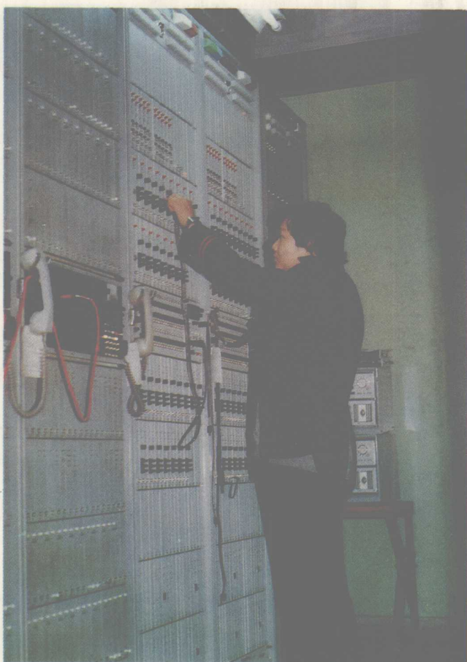
（左图）八十年代建成的 DD14 型和 JDD01-B 型长途半自动电话对端设备。
