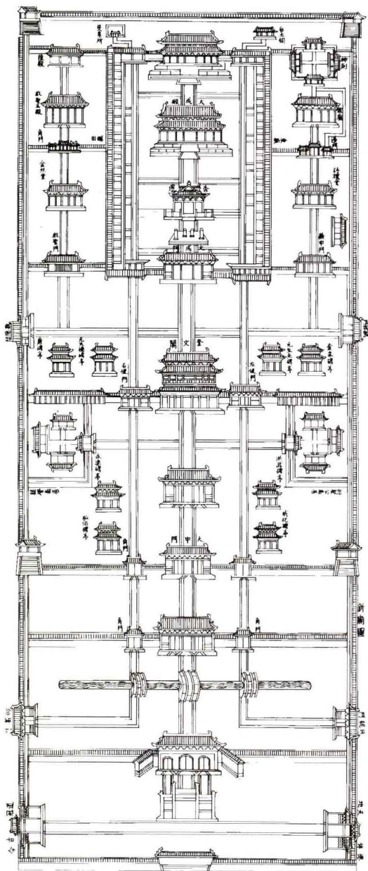
明代孔庙平面图
