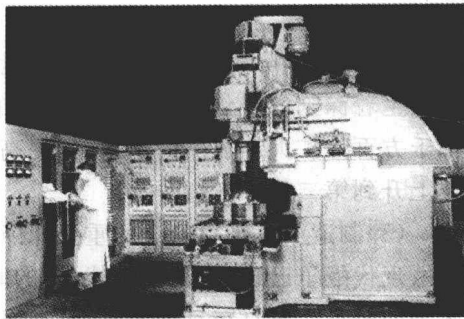
图 1-3 1952 年美国制造的数控机床
