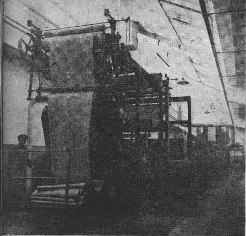
上漿拉幅烘燥聯合機正在操作
