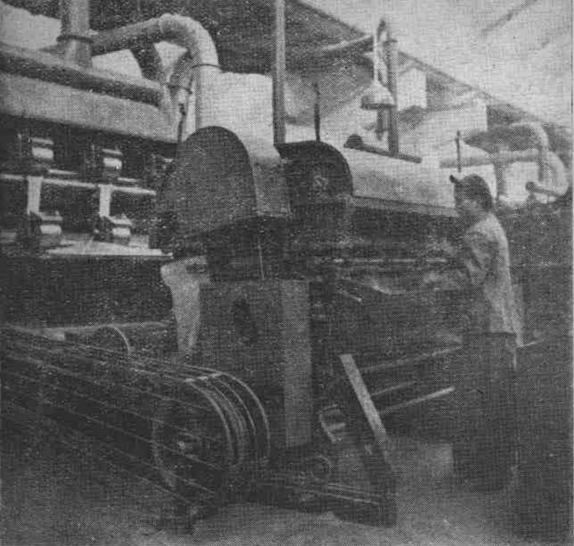
聯合梳麻機旁的安全保護設備
