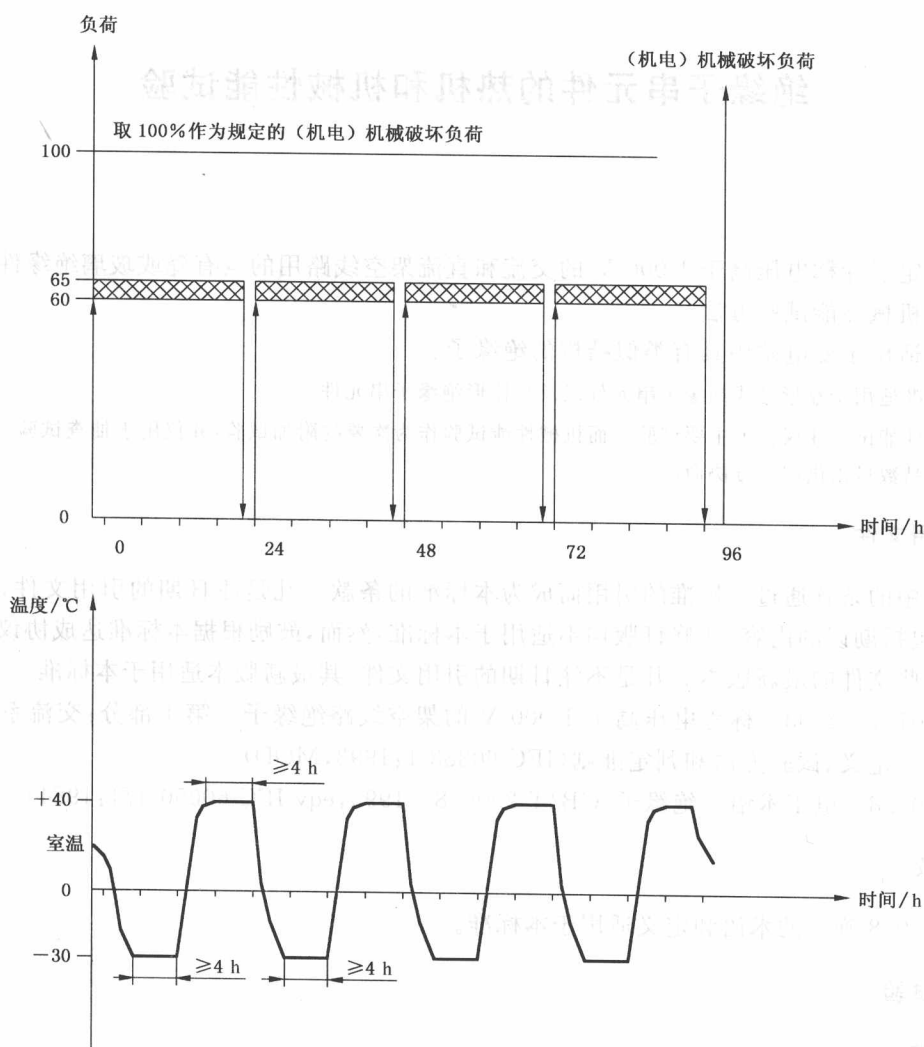
图 1 热机性能试验图示
