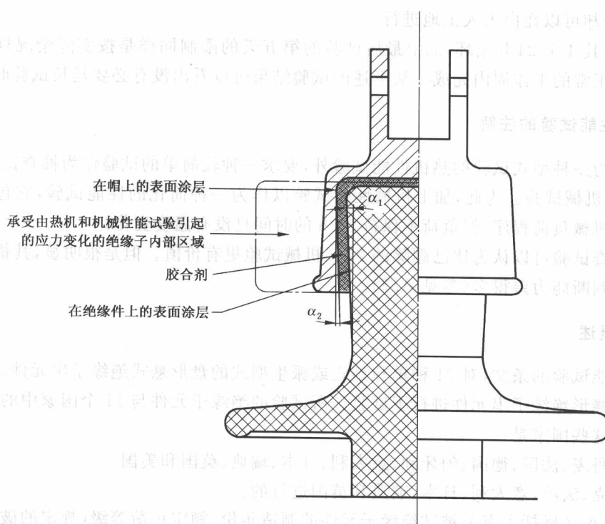
图 A.3 长棒形绝缘子横剖面
