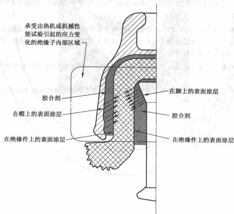
图 A.1 盘形悬式绝缘子的横剖面
