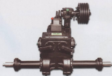
联合收割机变速箱
