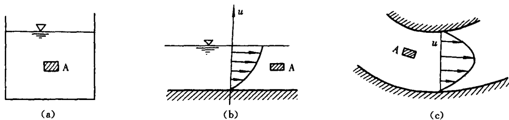
图 1-9 复习思考题 1-6 图
