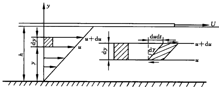
图 1-1 流体的粘性
