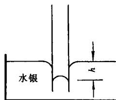
图 1-5 水银的毛细现象
