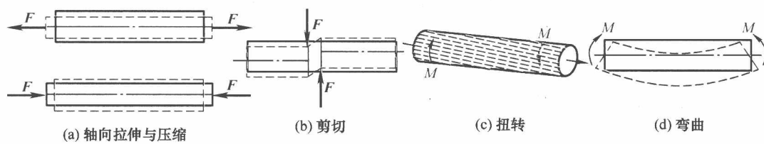
图 0-5 杆件的基本变形
