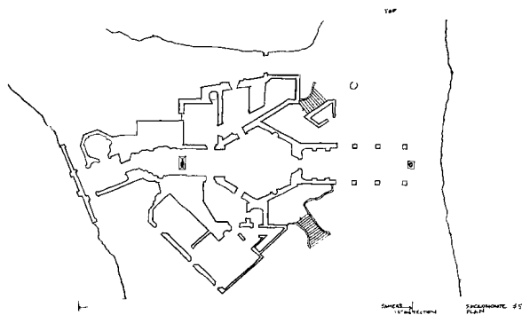
平面设计图，德·塞克罗门特，阿美卡美卡，墨西哥。
