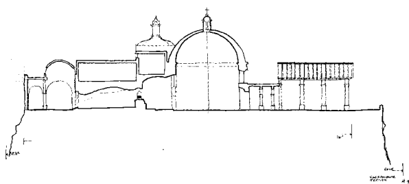
通过洞穴、地下室、避难所和门廊的剖面图。德·塞克罗门特，阿美卡美卡，墨西哥。
