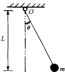
图 1-2 单摆
