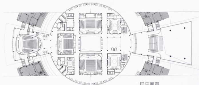
二层平面图
